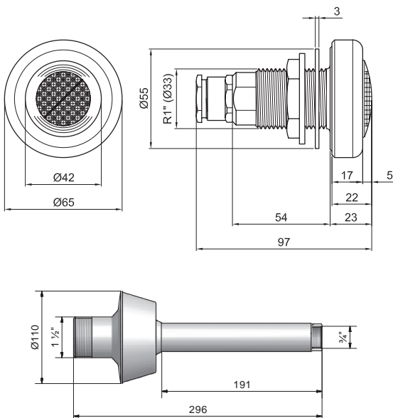
Non leak flange
